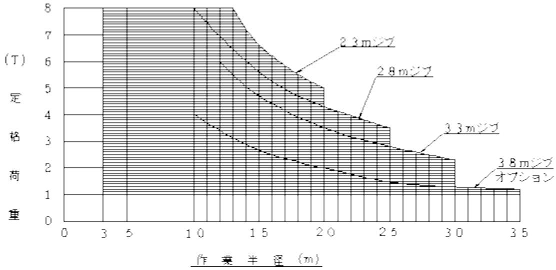
性能曲線図
