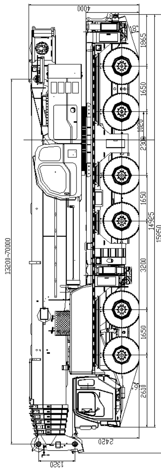
徐工 QAY260 型全地面起重机
