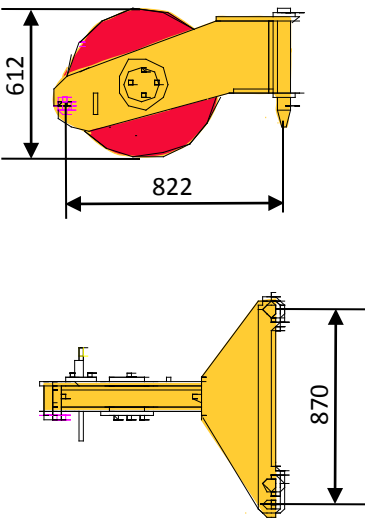
臂端单滑轮 107kg Single top
