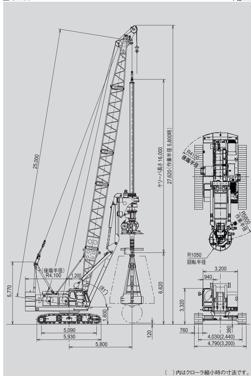
■寸法図
