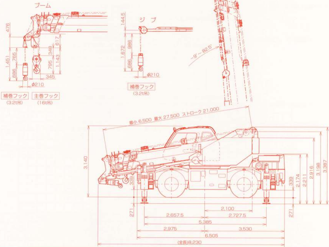
H型アウトリガ
